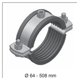
Rohrschelle Titan HD Seite 1/17
